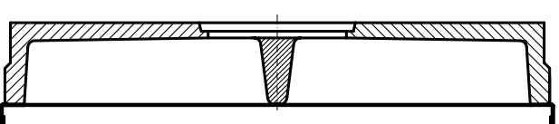
Schnitt C-C
